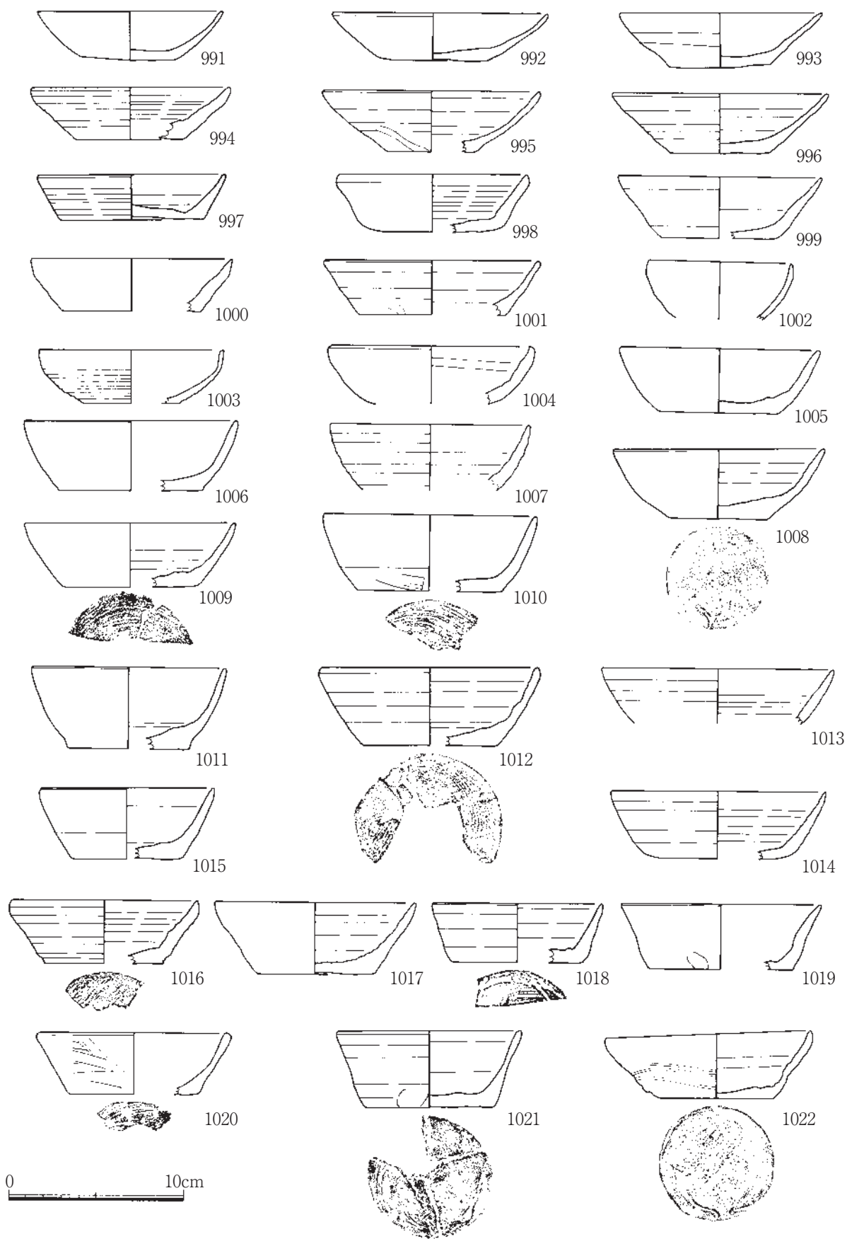
第70図 3A区遺物実測図3
