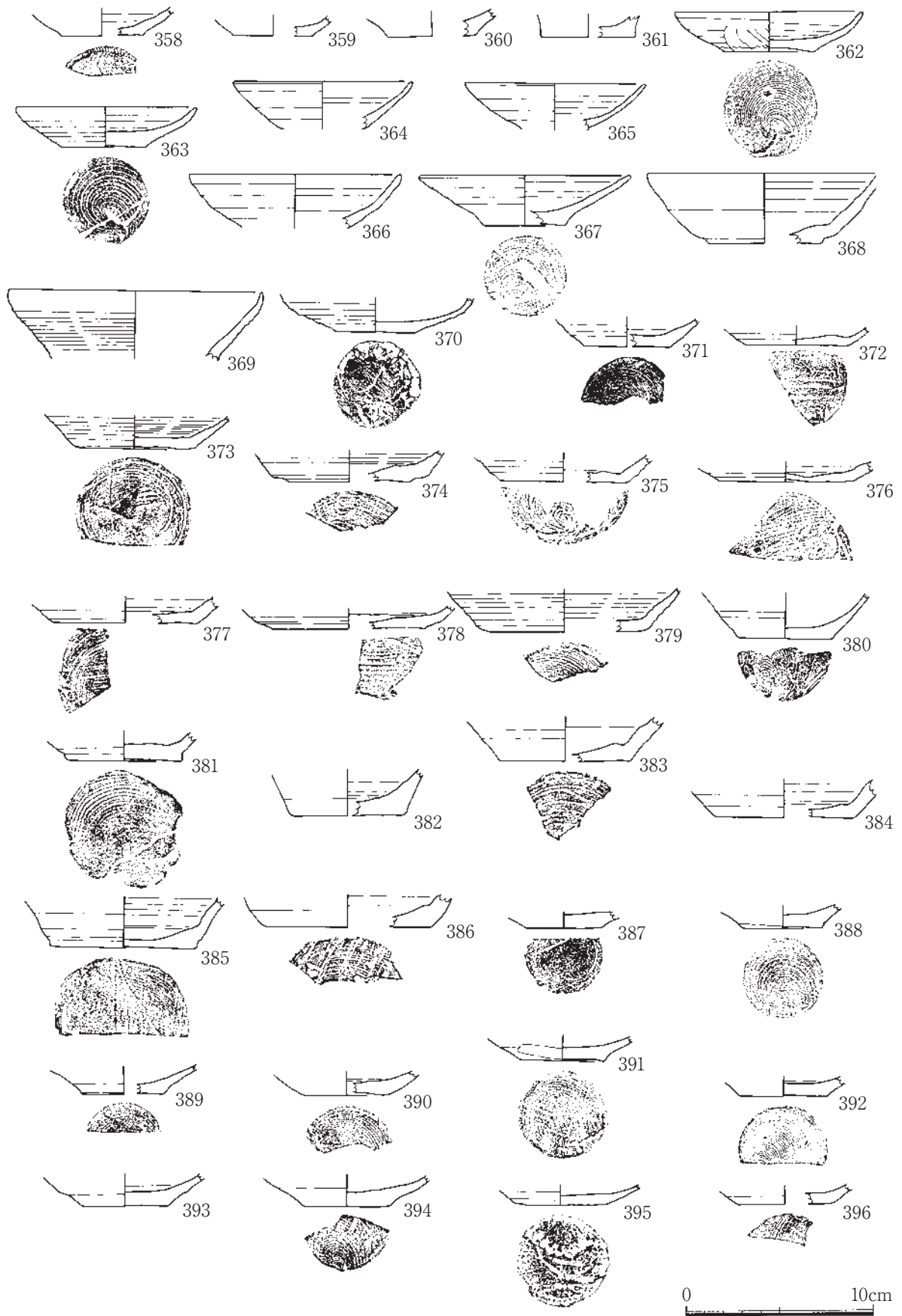
第28図 2A区遺物実測図6
