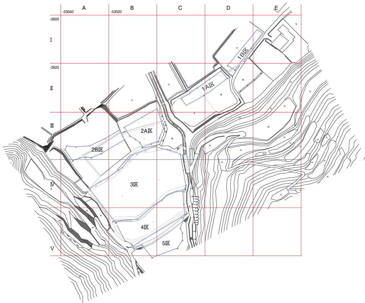
第4図 グリッド設定図
