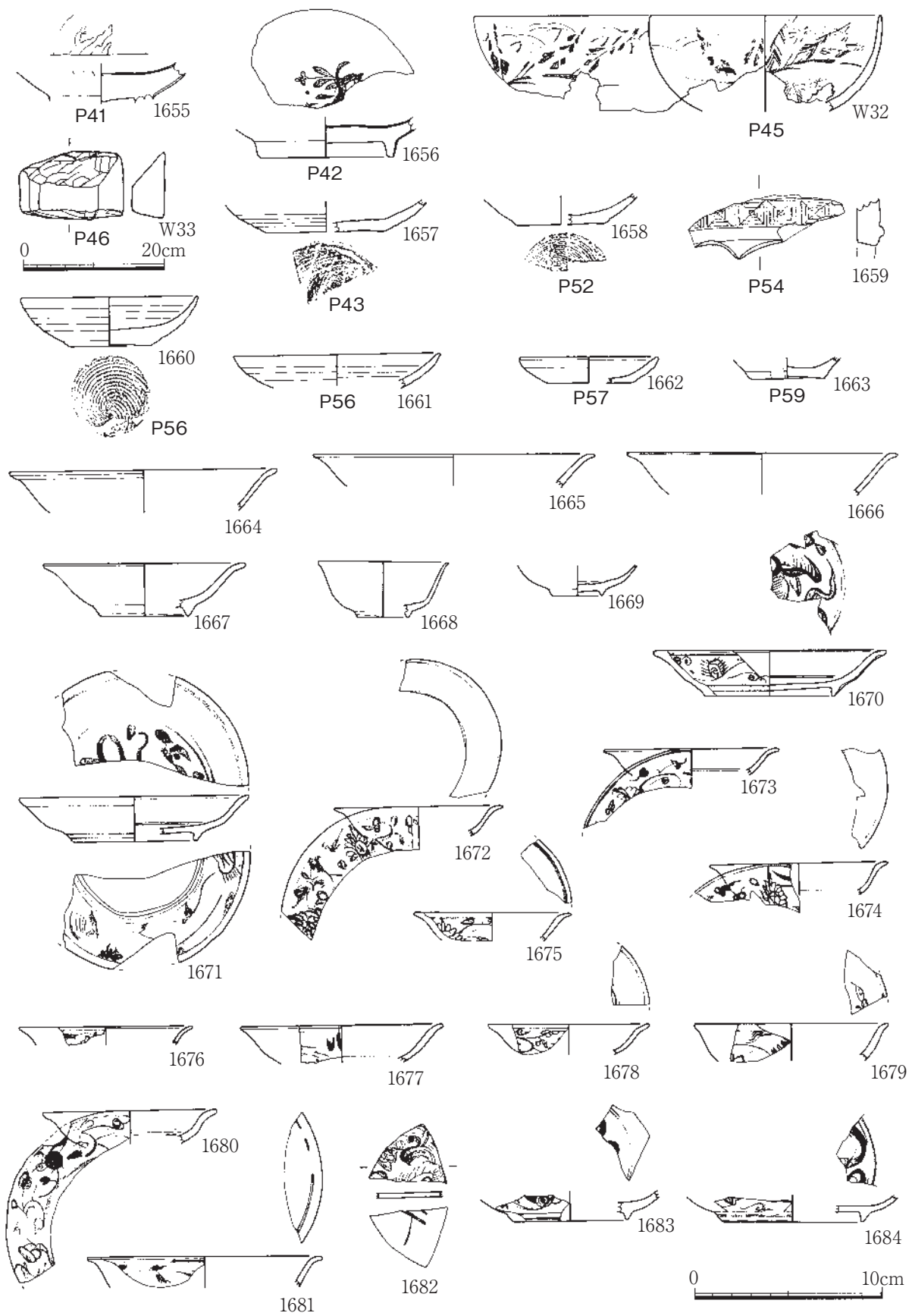
第104图 4区遺物実測図2
