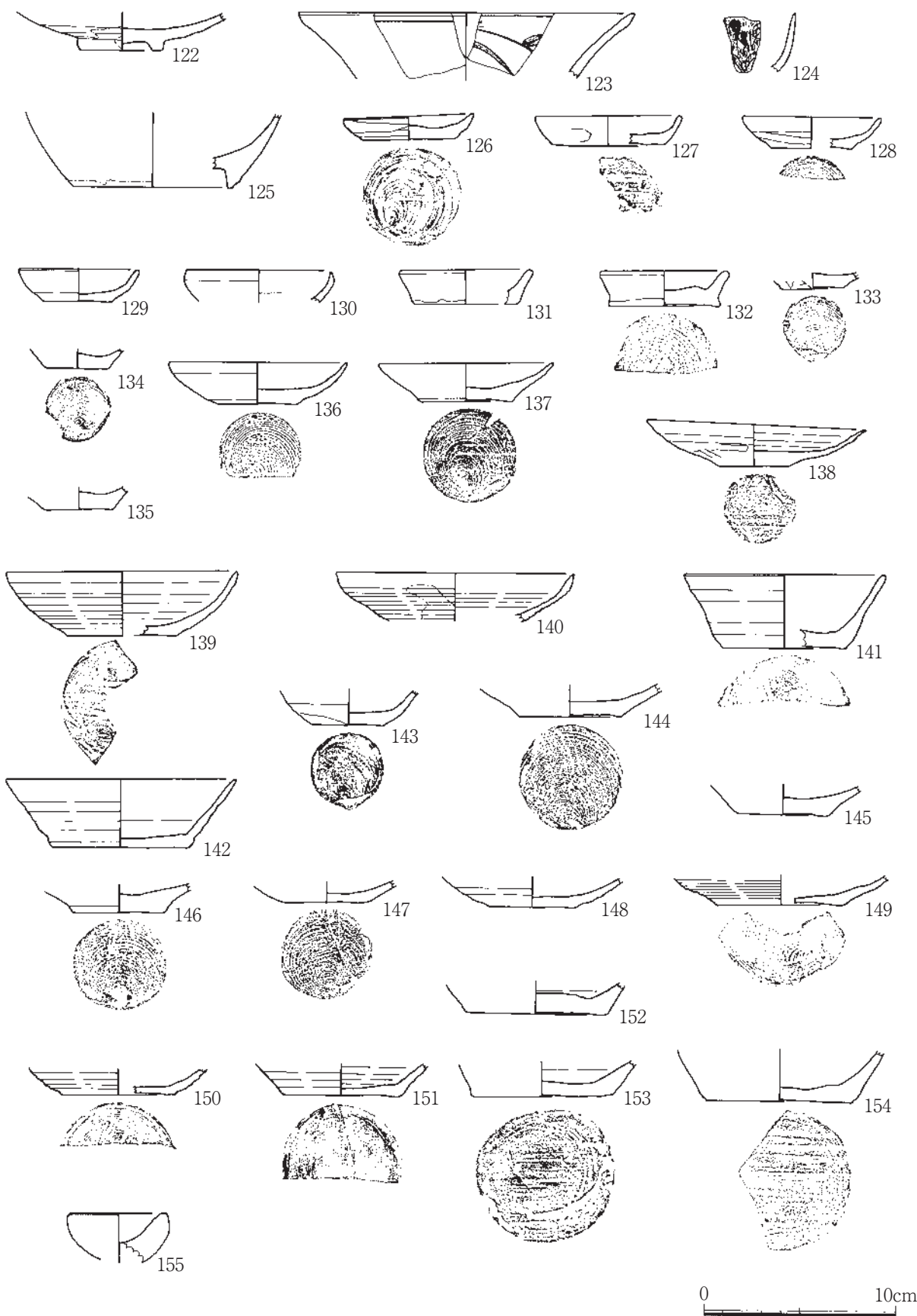
第17図 1B区遺物実測図2
