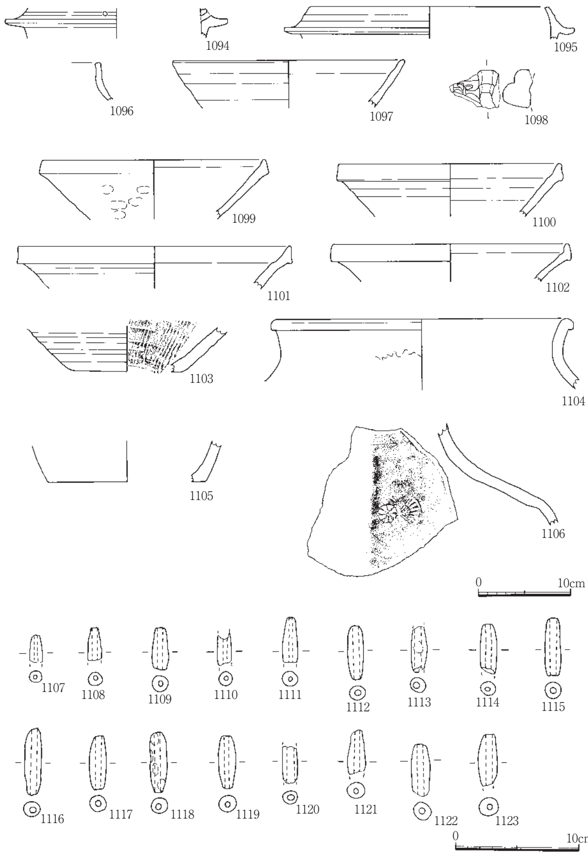
第73图 3A区遺物実測図6
