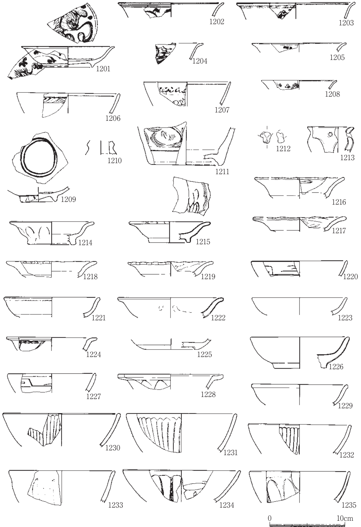
第81図 3B区遺物実測図1
