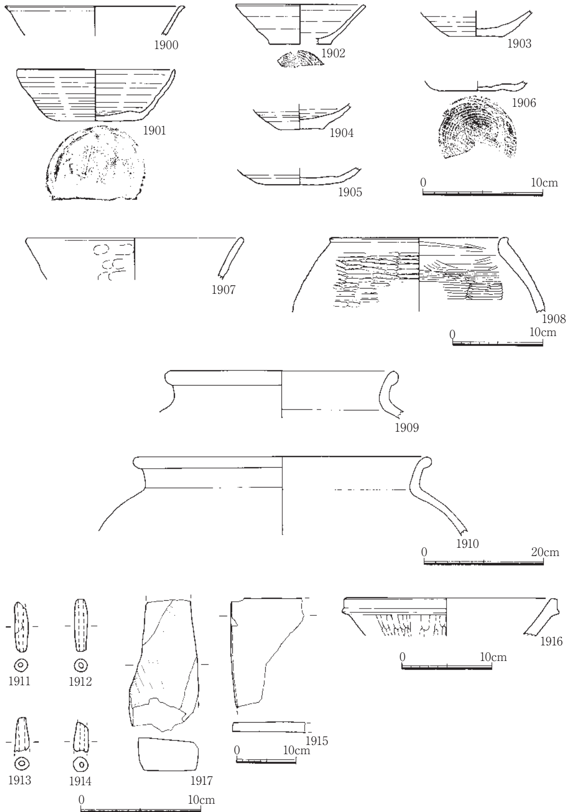
第116図 大溝2B区SD1遺物実測図
