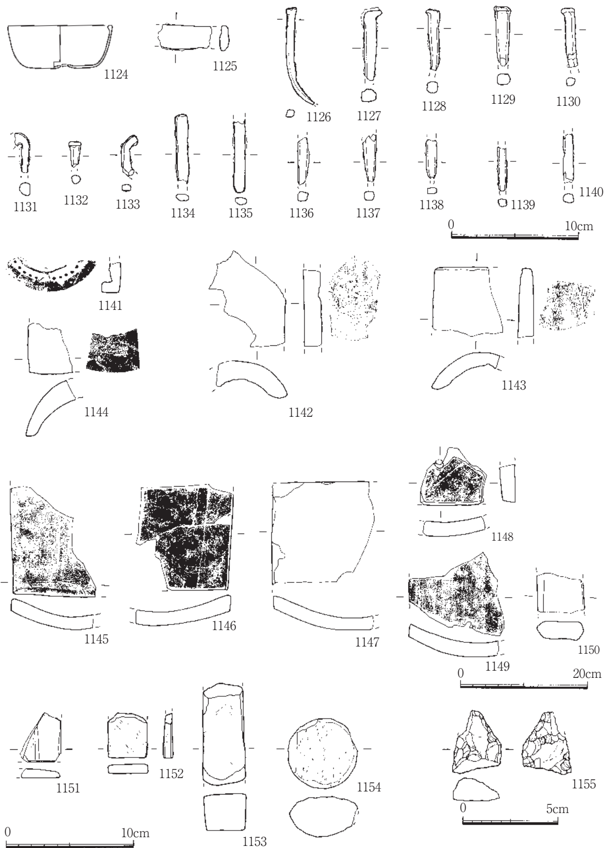
第74図 3A区遺物実測図7
