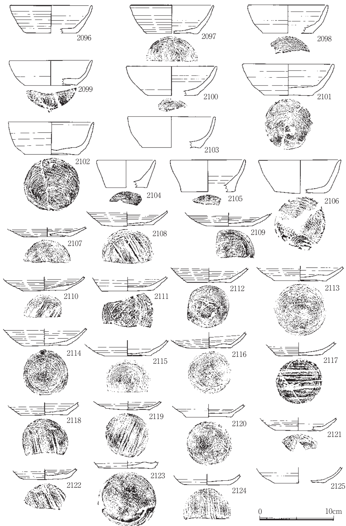
第122図 大溝SD1遺物実測図6
