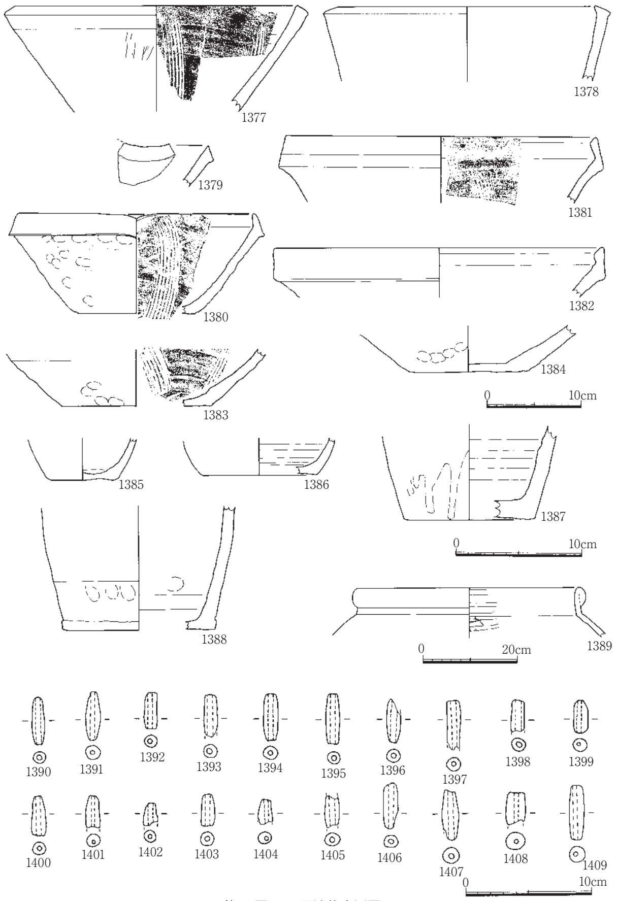
第86图 3B区遺物実測図6
