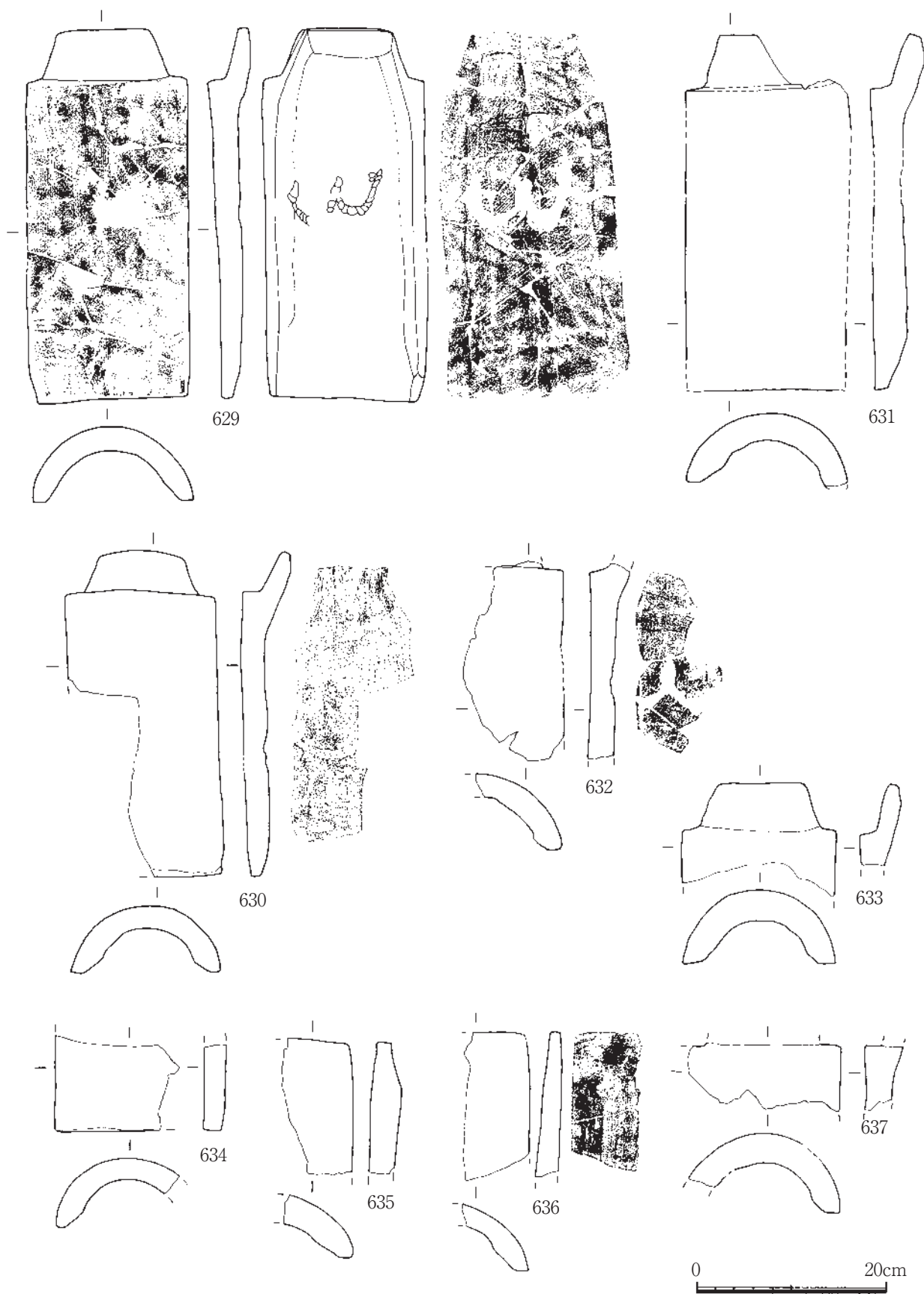
第55図 2号瓦窯遺物実測図2
