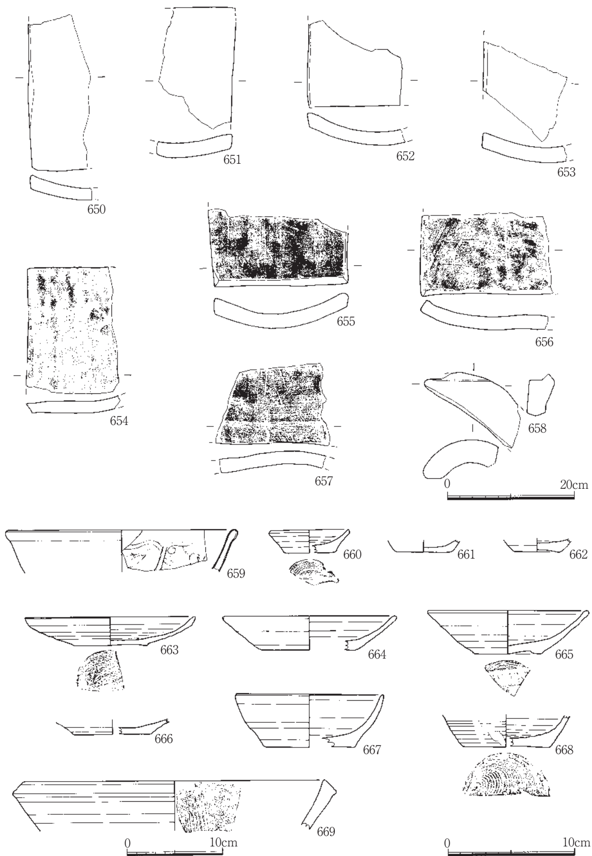
第57図 2号瓦窯遺物実測図4
