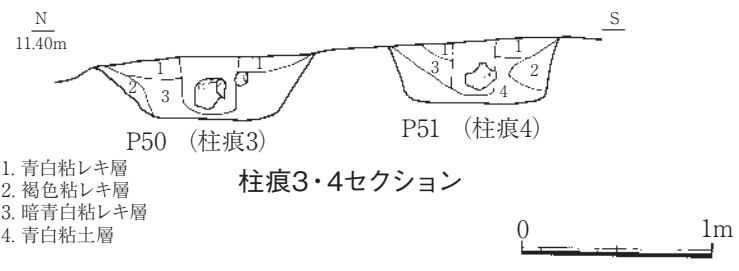
第101図 4区柱痕1～4
