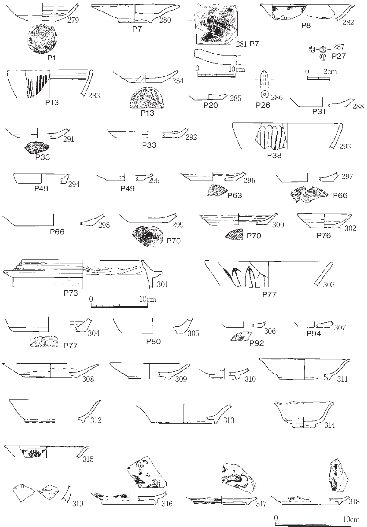
第26図 2A区遺物実測図4
