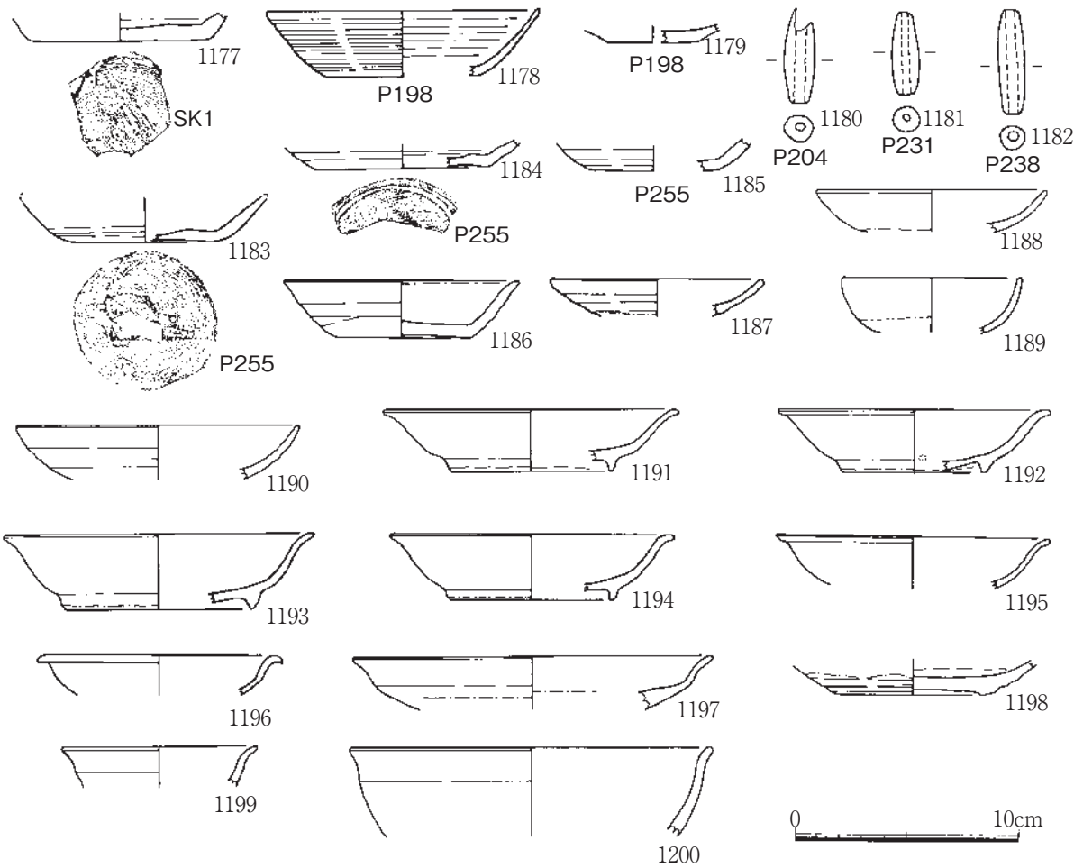
第80図 3B区瓦溜り2・土坑・柱穴遺物実測図
