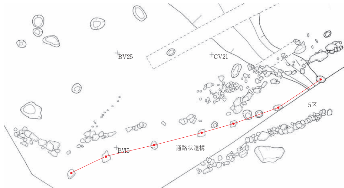
第102図 4区通路状遺構
