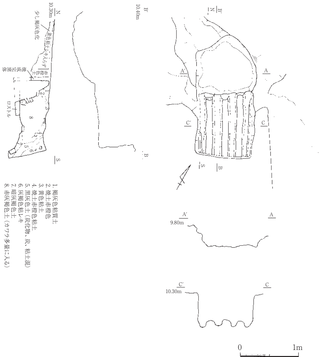
第47図 1号瓦窯
