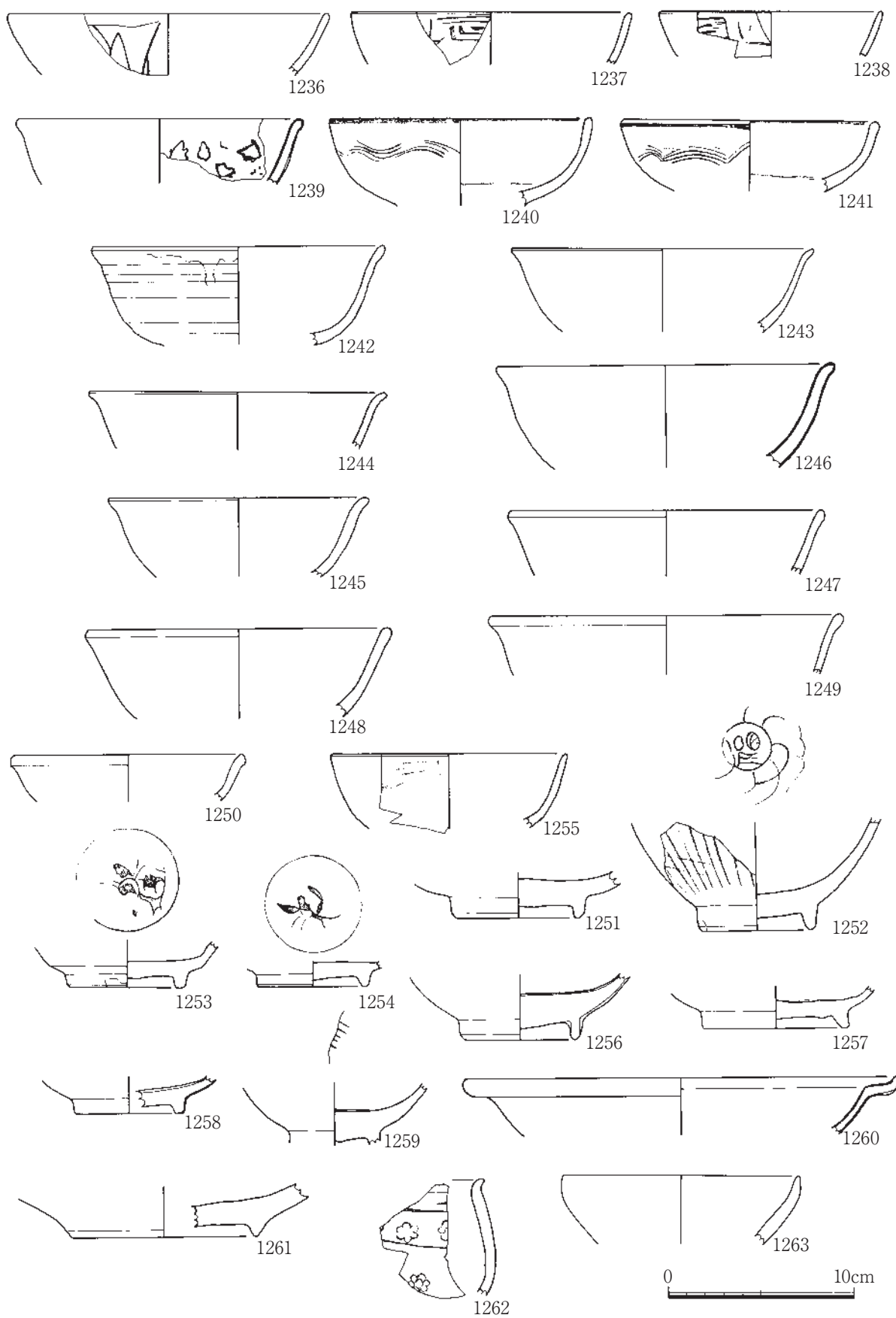
第82図 3B区遺物実測図2
