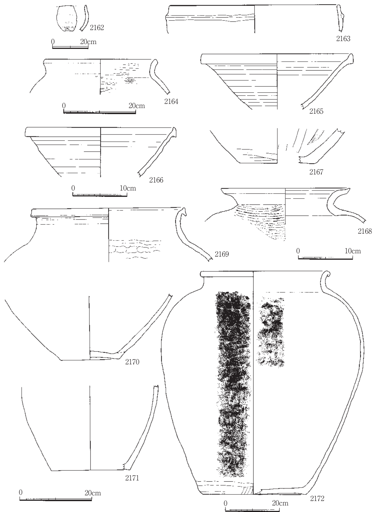
第124図 大溝SD1遺物実測図8
