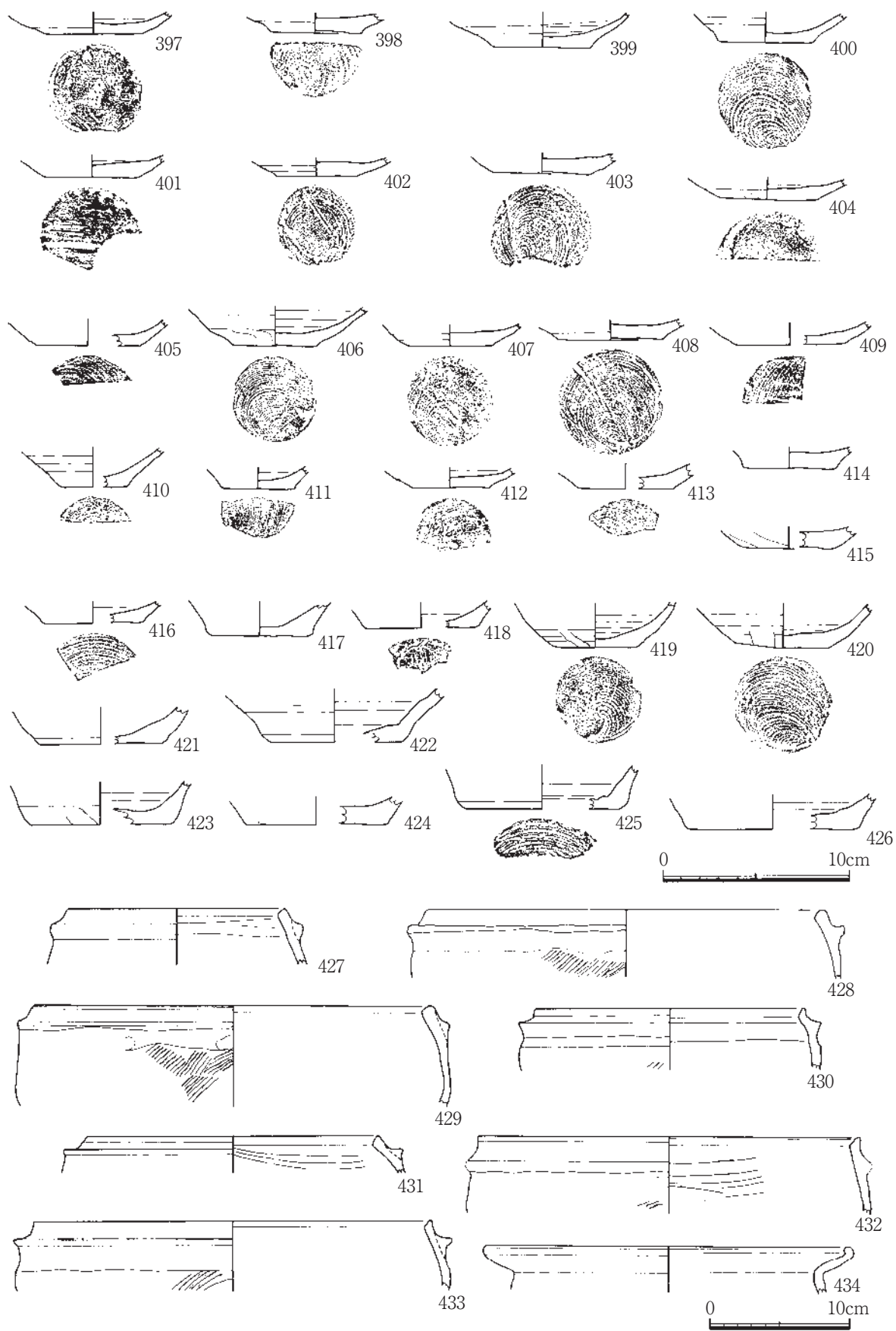
第29图 2A区遺物実測図7
