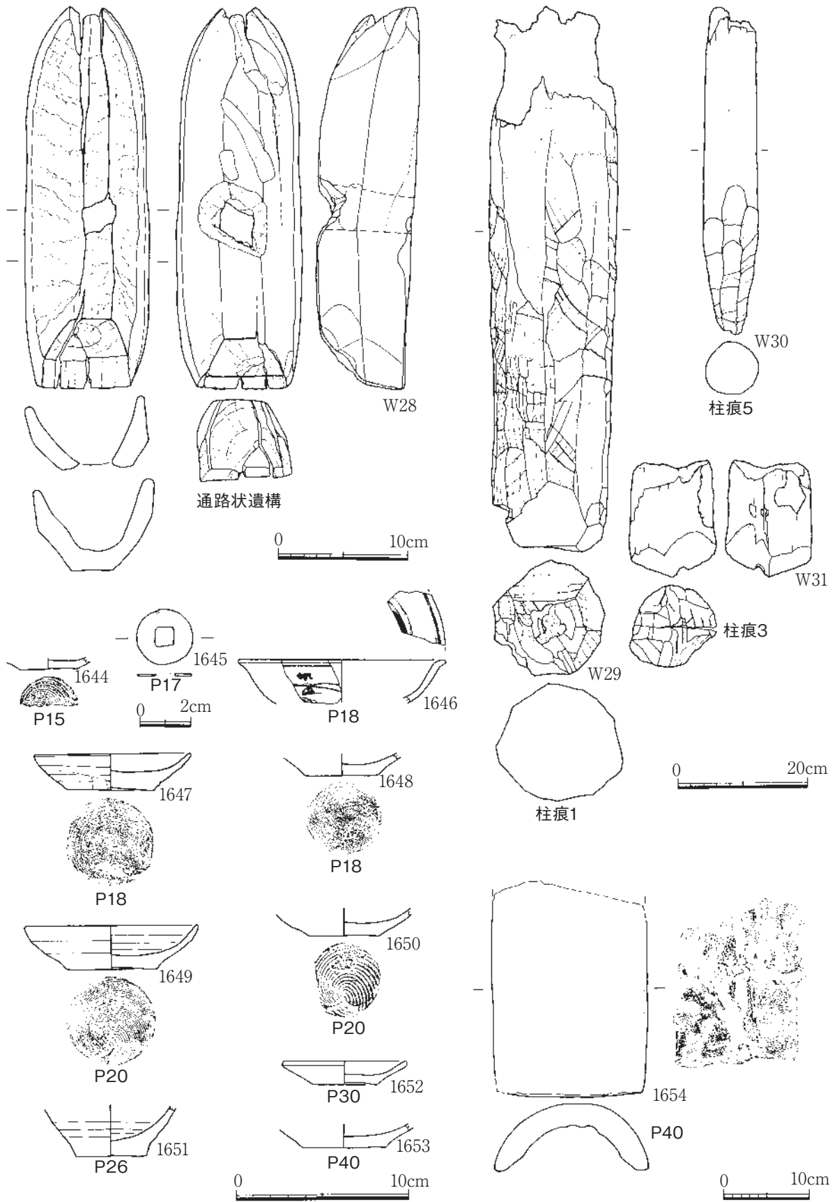
第103図 4区遺物実測図1
